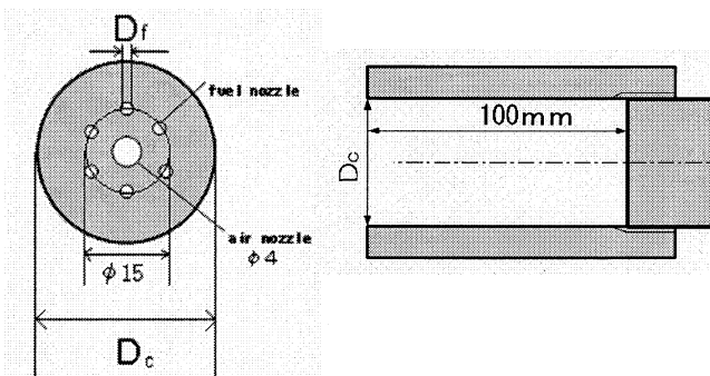
図 1 ノズル配置と燃焼室
