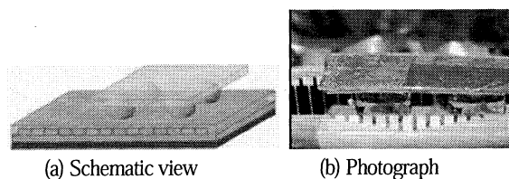
Fig. 14 Linear actuator
