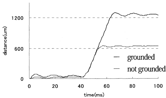
Fig. 9 Droplet motion
