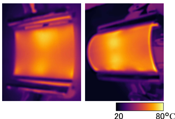
図2 透明導電性フィルム(5×5 cm 2 )に30 V印加した時のサーモグラフィー
