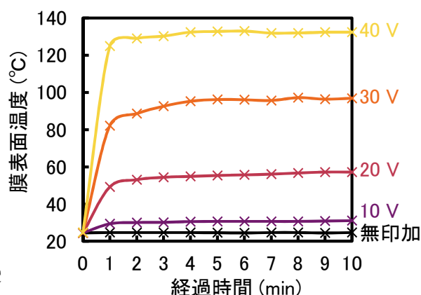
図3 透明導電性フィルム(5×5 cm 2 )に各電圧を印加したときの表面温度
