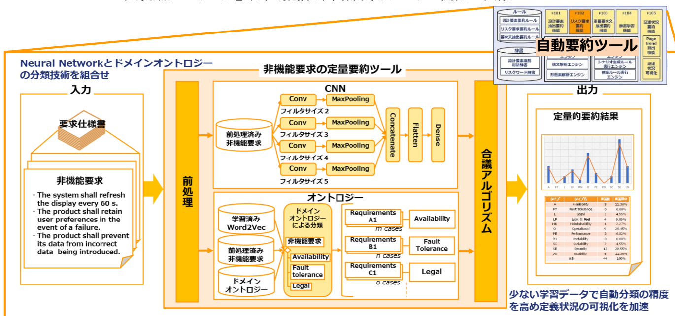
図1 CNNとドメインオントロジーの分類技術を組合せた非機能要求の定量化自動要約の仕組み
